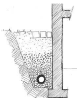
B - Réalisation d'un drainage périphérique de la construction en l'absence ou en complément d'une gouttière.
